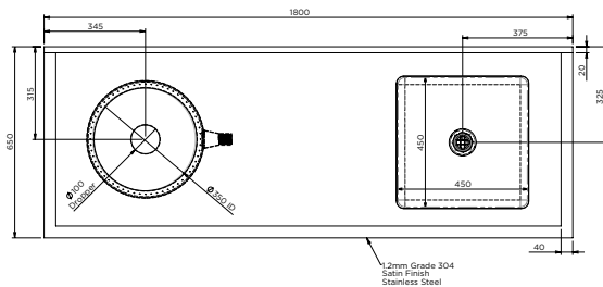
MODEL LDUS-A Plan
