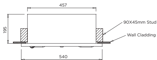
MODEL DIWR Plan
