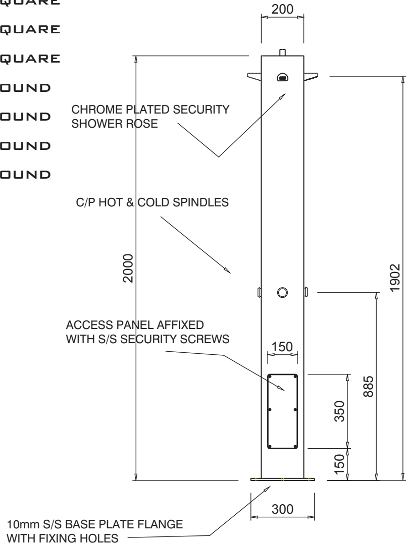
ELEVATION - CSS4
