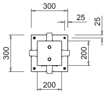
PLAN - CSS4
